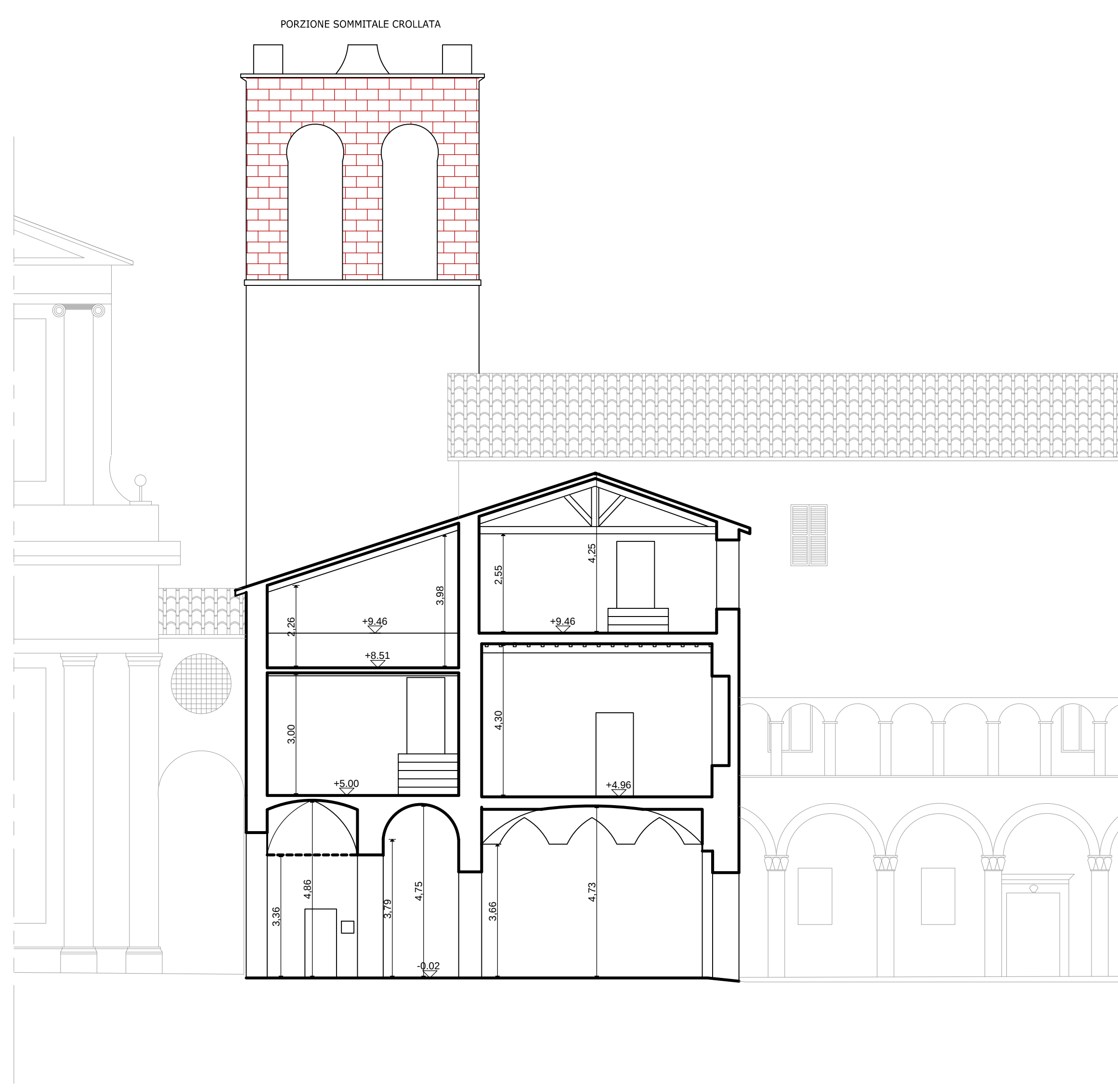
sezione 3-3
