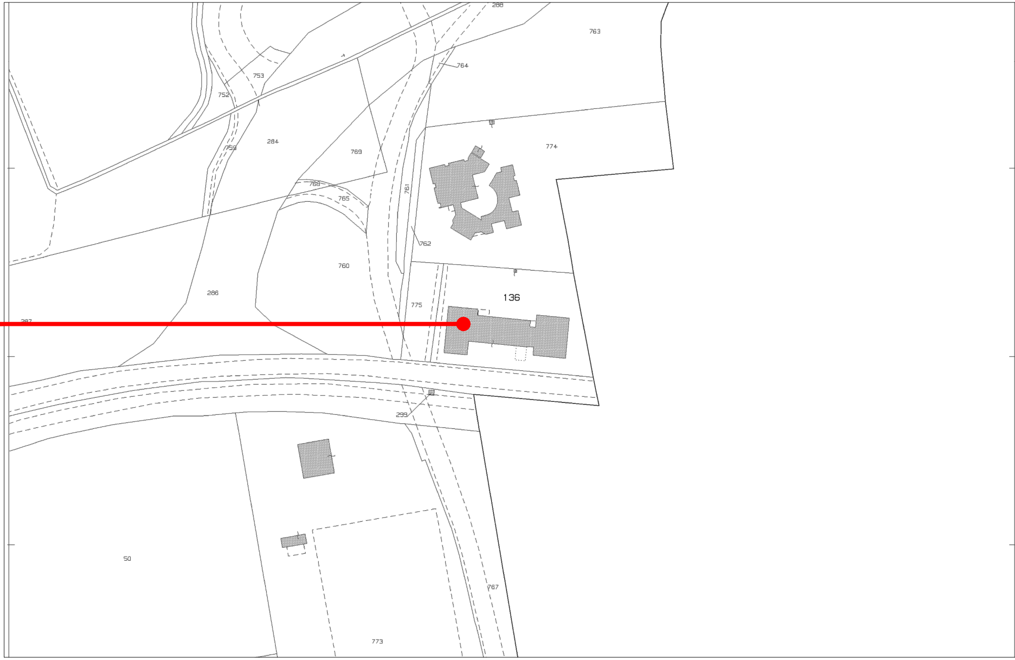
Stralcio Planimetria Catastale - Fig.159 Part. 136
