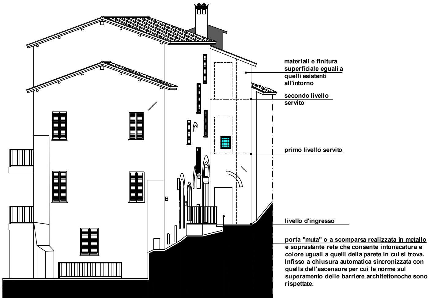
PROSPETTO FRONTALE
